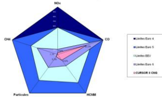
Emissions Moteur CURSOR 8 CNG sur cycles ETC
