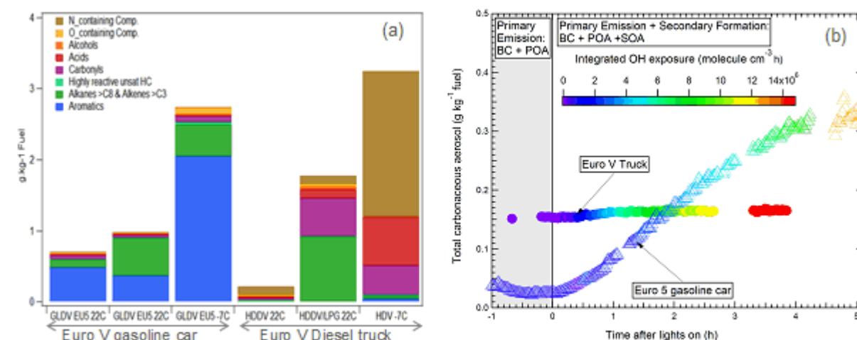
Légende de la Figure : (a) composition globale de la phase gazeuse telle que vue par le PTR-MS pour les émissions primaires du véhicule léger essence Euro 5 (Fiat 500) et du camion Euro 5, (b) vieillissement comparé de l'aérosol émis par le véhicule léger essence Euro 5 et le camion Euro 5 Diesel – le code couleur représente la quantité intégrée d'exposition à OH : les émissions du véhicule essence sont très réactives (consommation importante de OH), les émissions du véhicule Diesel sont moins réactives (consommation plus faible des OH)
